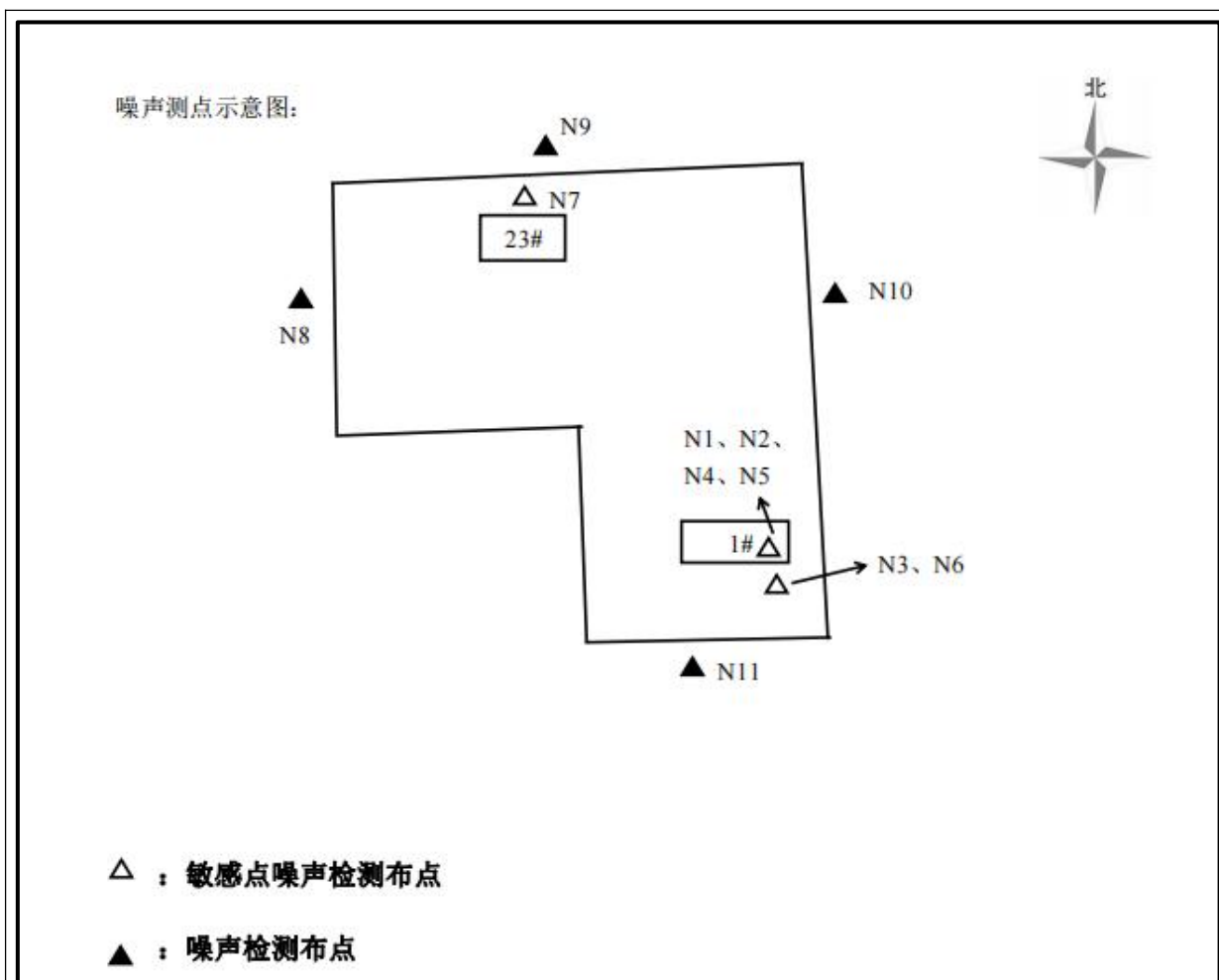
图 6-1 噪声测点示意图
